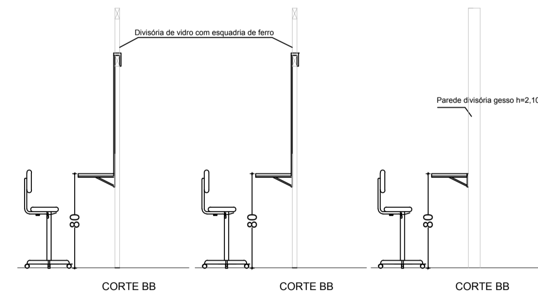
CORTE BB
