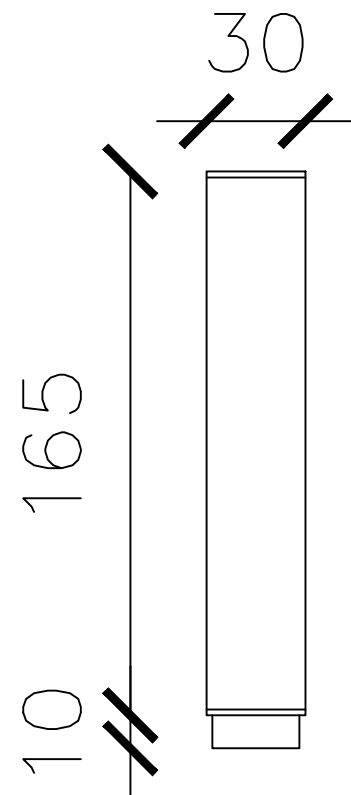
VISTA LATERAL
