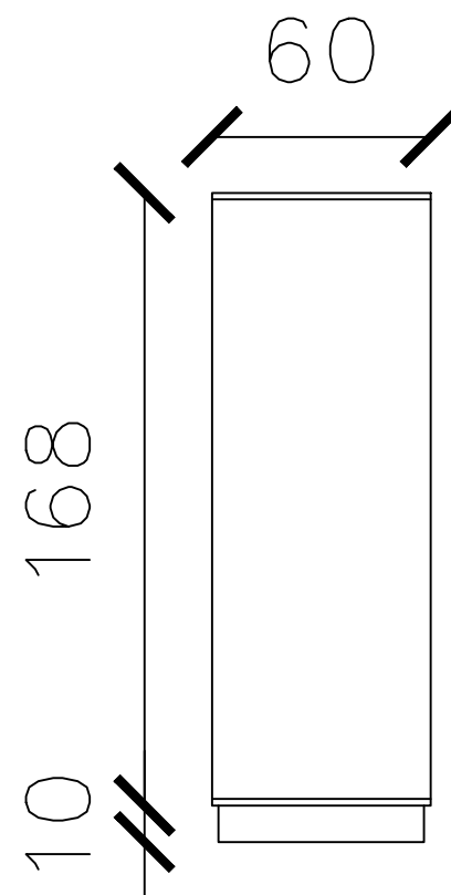
VISTA LATERAL
