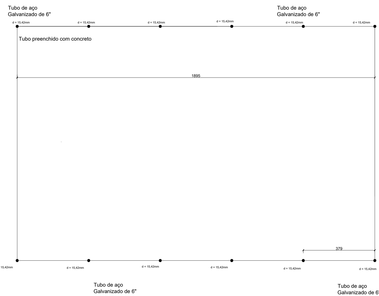
Localção de Pilares h = 4,50m
